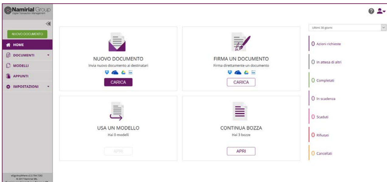
Figura 1 - GUI eSAW
